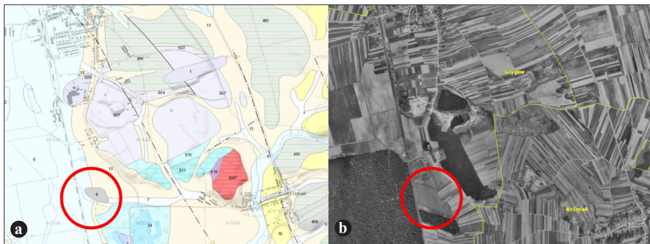
Obr. 6. Odhadovaná typová lokalita ostřice Otrubovy u obce Grygov. Podkladové mapy: a) geovědní mapa 1:50 000 s vyznačením slatin východně lesa Království. – © ČGS; b) letecký snímek z roku 1954. – © Národní geoportál INSPIRE
